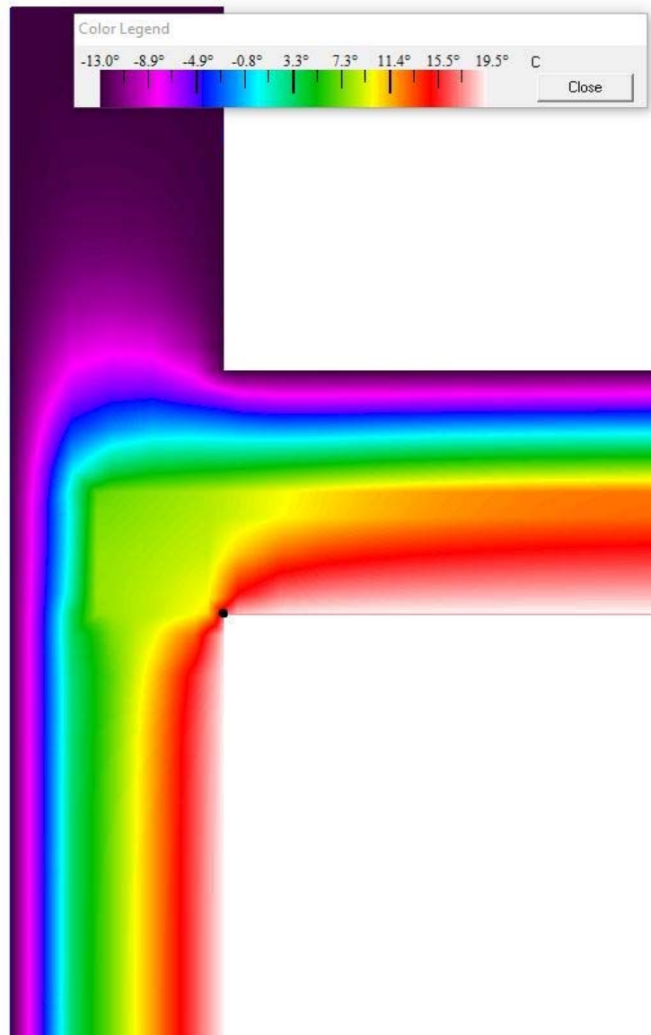
Priebeh teplôt konštrukciou - vykreslenie pomocou teplotného poľa
