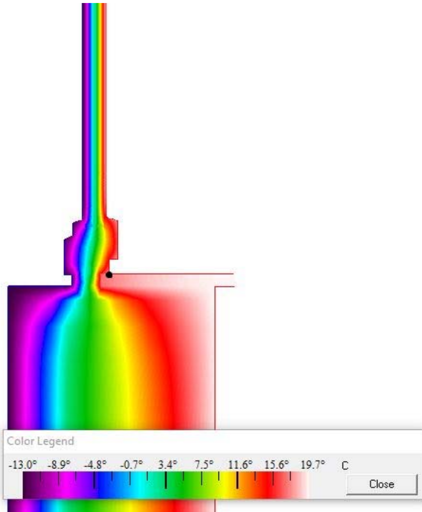
Pribeh teplôt konštrukciou - vykreslenie pomocou teplotného poľa
