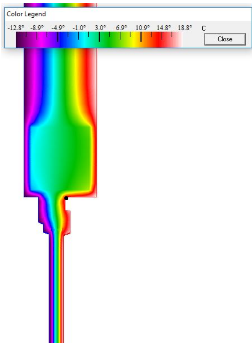
Priebeh teplôt konštrukciou - vykreslenie pomocou teplotného poľa
