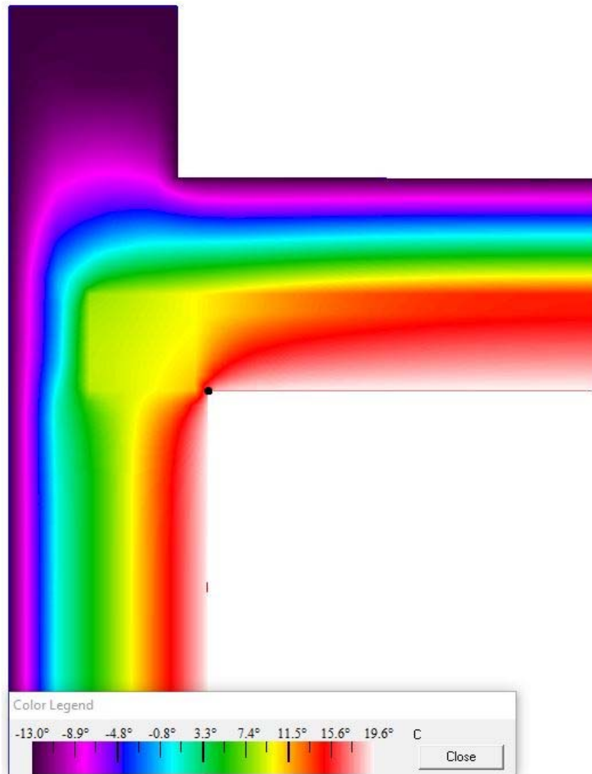
Pribeh teplôt konštrukciu - vykreslenie pomocou teplotného poľa
