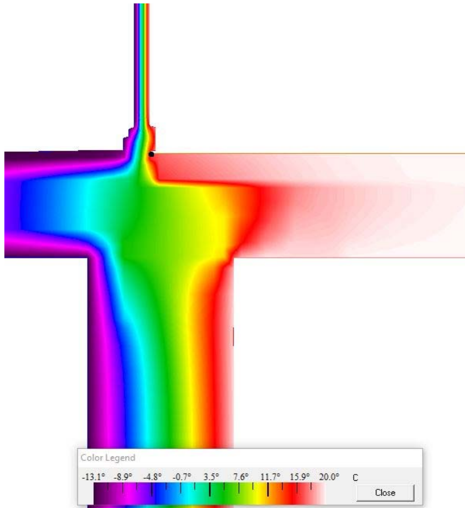
Pribeh teplôt konštrukciou - vykreslenie pomocou teplotného poľa
